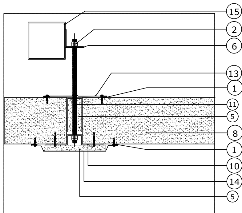
SECTION A-A
